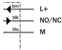
3 x 0.15 mm 2
